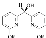
171a: OR=(1 S ,2 R ,5 R )-isomenthoxy1 171b: OR=(1 S ,2 R ,4 S )-borneoxy1
