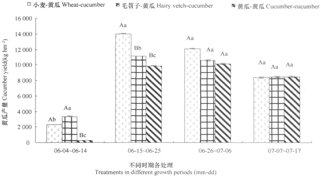
图 6 不同轮作处理对不同时期黄瓜产量的影响
