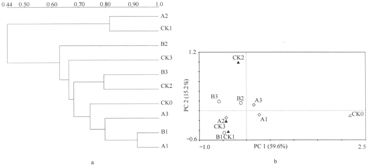
图 2 不同轮作处理各时期土壤细菌群落相似性分析 (UPGMA) (a)及主成分分析 (b)
