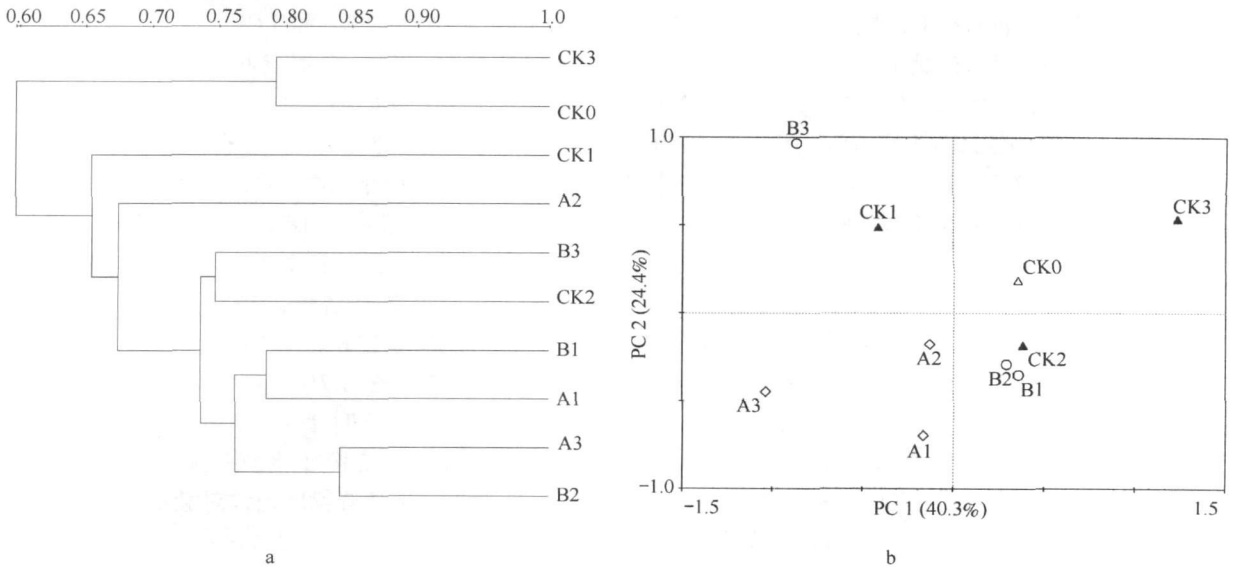
图 4 不同轮作处理各时期土壤真菌群落相似性分析 (UPGMA) (a) 及主成分分析(b)
