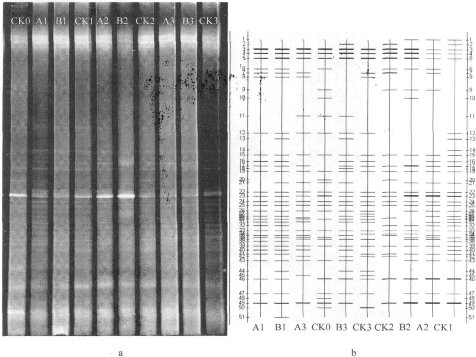
图1 不同轮作处理各时期土壤细菌 DGGE图谱 (a) 及泳道/条带识别图 (b)
