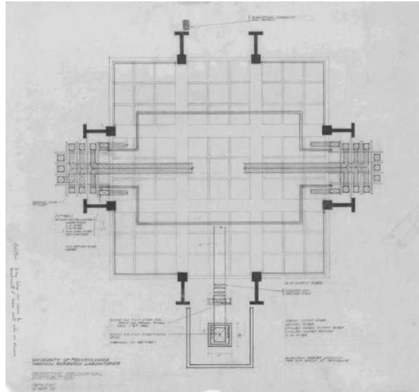
Fig. 2 Diseño del paso de las instalaciones entre las vigas hasta los espacios servidores. Croquis del despacho de LIK. Nro. Lámina 430. IC.490.1.2. The A. A., U. of Penn.
