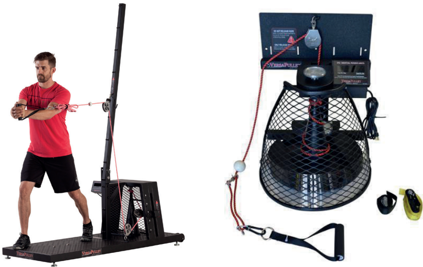
Figura 33. Versapulley tipo de dispositivo para ejercicio Inercial
