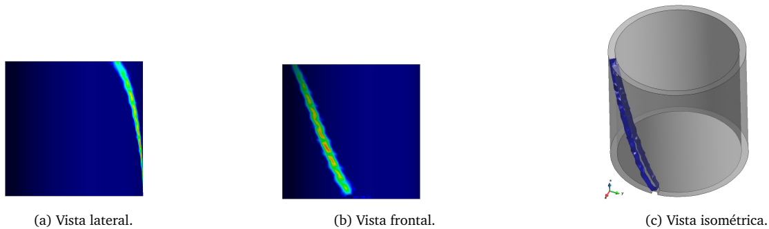
Figura 15: Deformaciones plásticas equivalentes en el modelo de MC con \phi = 45^\circ en torsión pura. Ángulo de localización teórico: \theta_{loc}^{teo} = 22.5^\circ con el eje vertical ( 67.5^\circ con el plano horizontal). Ángulo de localización numérico: \theta_{loc}^{num} = 22.47^\circ .
