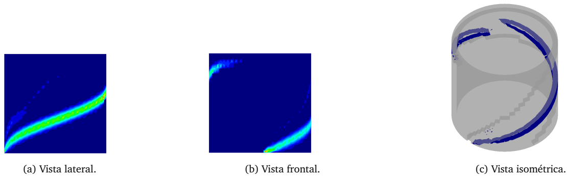
Figura 14: Deformaciones plásticas equivalentes en el modelo de MC con \phi = 45^\circ en torsión con perturbación de tracción. Ángulo de localización teórico: \theta_{loc}^{teo} = 22.5^\circ con el eje horizontal. Ángulo de localización numérico: \theta_{loc}^{num} = 23.62^\circ .
