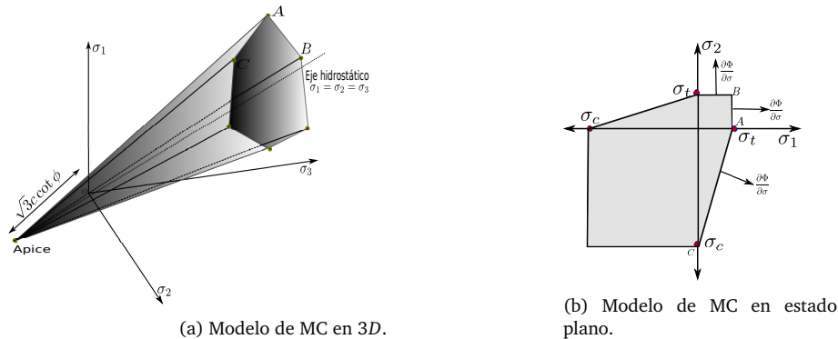
Figura 1: Modelo de Mohr-Coulomb.
