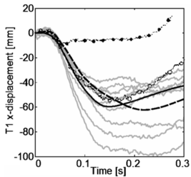
-- Hybrid III, — BioRID P3, -- TNO, — Mode
