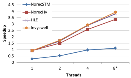
(g) ssca2.
