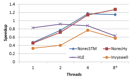
(j) Yada.
