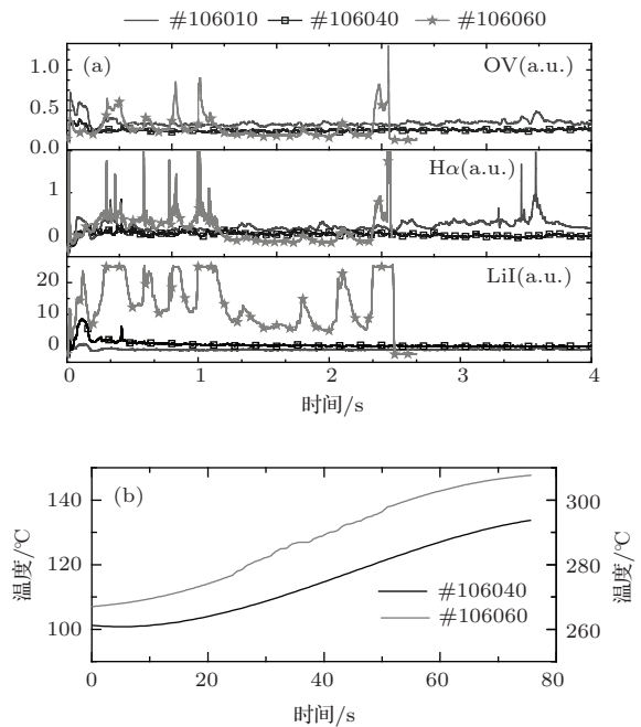
图3 不同放电条件下的参数 (a) 不同放电条件下 OV, H \alpha , LiI 的相互比较; (b) 第 106040 和 106060 次放电点下限制器温度随时间的变化曲线
