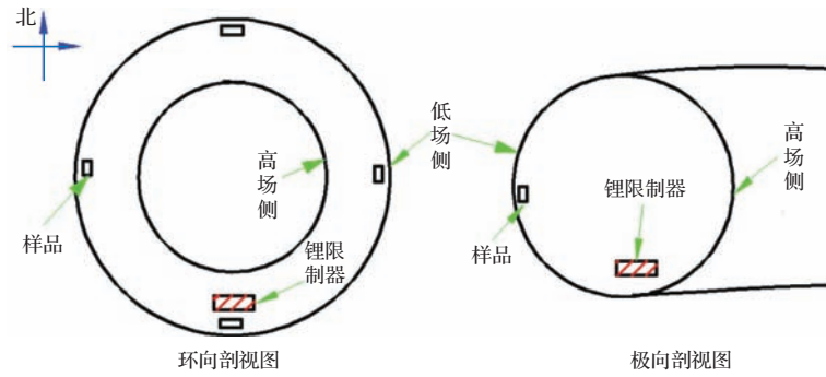
图2 锂限制器及样品的分布
