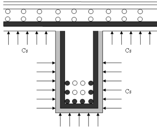
Figure 4: Schéma des armatures touchées par la corrosion due à la présence de sels déglçants en surface ( C_s )
