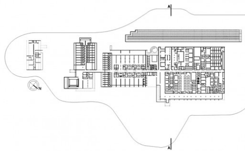
Planta térreo
