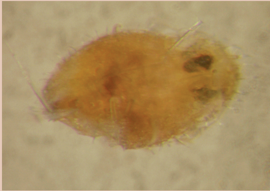
Figura 4. Pupario luego de la emergencia del parasitoide Encarsia sp. en ninfa de tercer estadio ninfal de T. vaporariorum . Por: Suárez, L., 2009.
