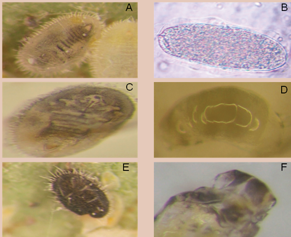
Figura 5. Diferentes estados de Encarsia formosa . A. Ninfa parasitada con el parasitoide en estado de huevo en contraste con una ninfa no parasitada (observar cambios de la pigmentación). B. Huevo de E. formosa . C. Ninfa parasitada con el parasitoide en estado de pupa . D. Larva de E. formosa . E. Ninfa parasitada con el parasitoide en estado de pupa. F. Pupa de E. formosa luego de la disección .Por: Suárez, L 2009.
