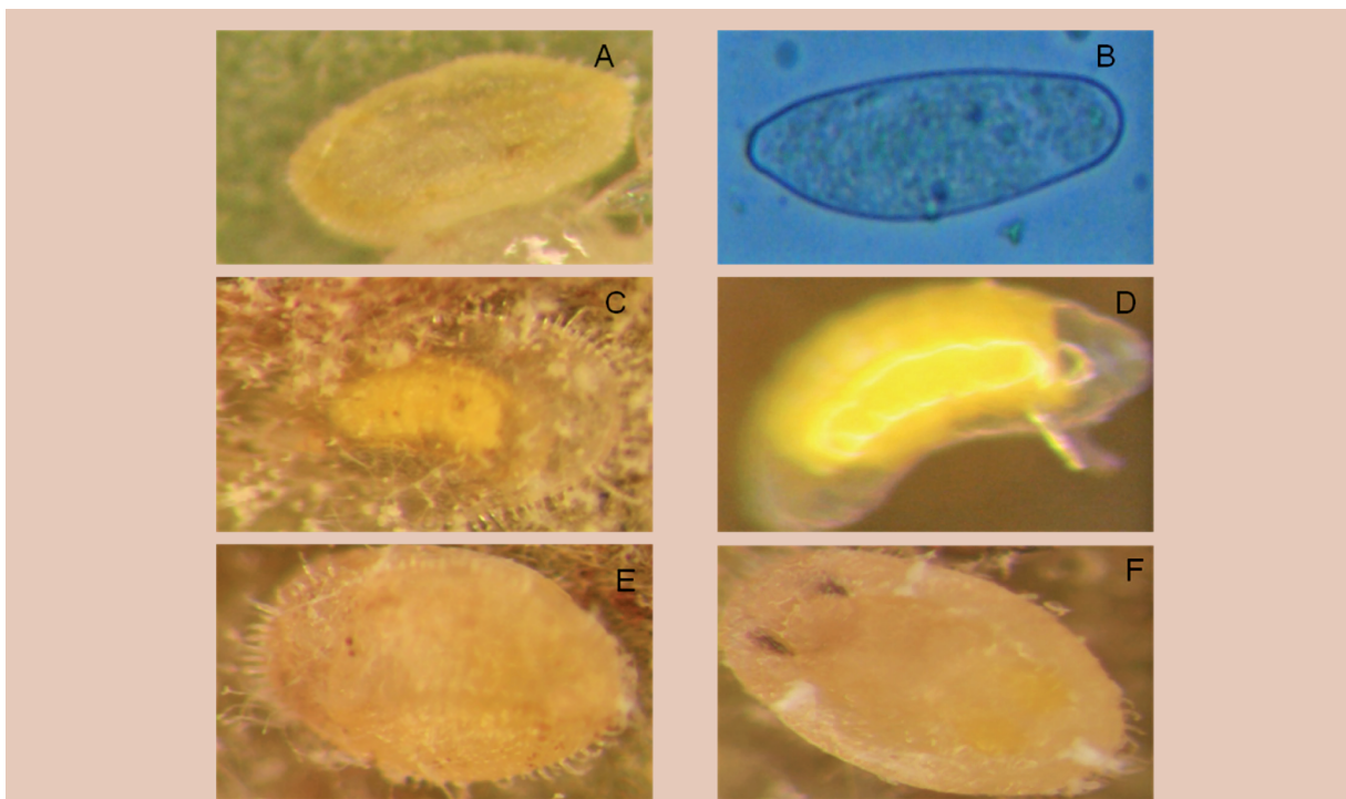
Figura 3. Diferentes estados de Encarsia sp. A. Ninfa parasitada con el parasitoide en estado de huevo. B.Huevo de Encarsia sp. C. Ninfa con vista de larva del parasitoide (10x). D. Larva. E. Ninfa parasitada con el parasitoide en estado de pupa (posición dorsal). F. Ninfa parasitada con el parasitoide en estado de pupa (posición ventral). Por: Suárez., L 2009.
