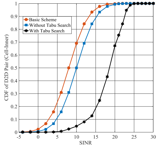
Fig. 3. SINR of D2D pairs in the inner cell region
