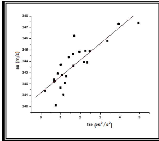
الشكل(5). العلاقة بين سرعة الصوت في الهواء Ss (m/s) والطاقة الحركية المضطربة tke (m^2/s^2)
