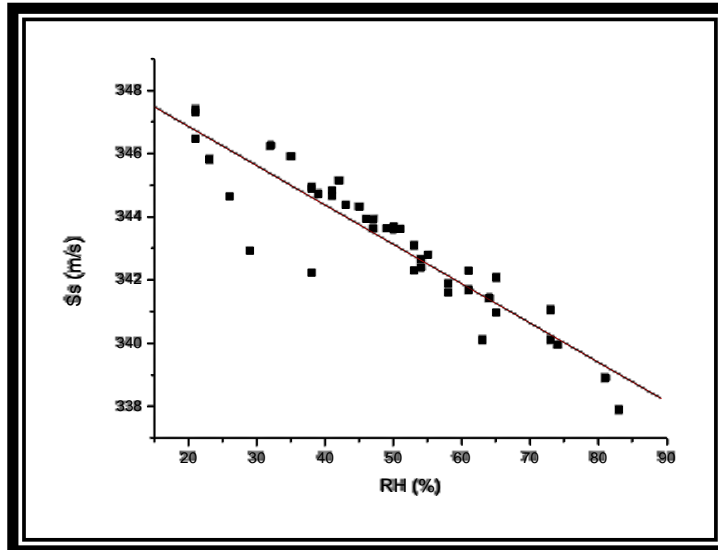
شكل (4). العلاقة بين سرعة الصوت في الهواء Ss والرطوبة النسبية للهواء RH
