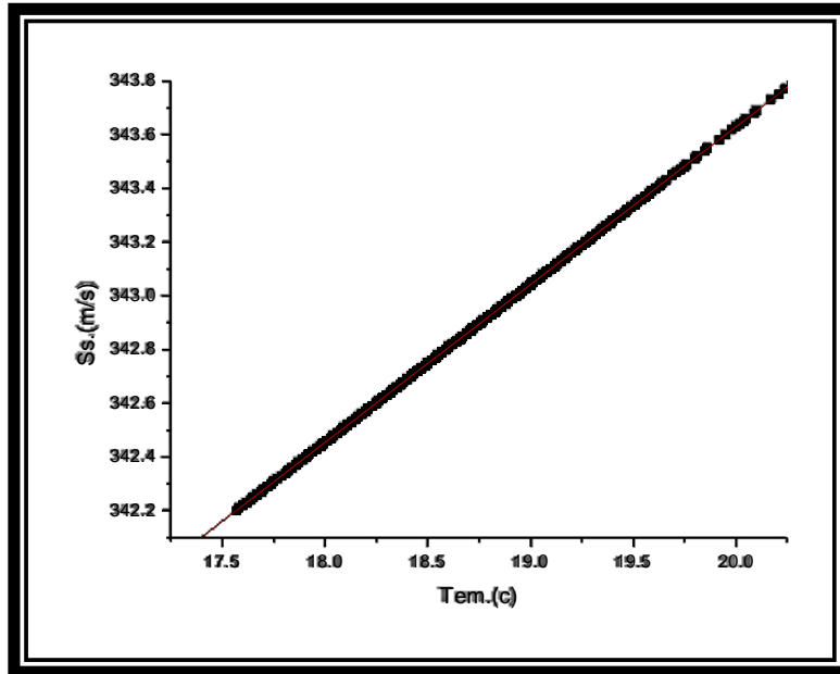
الشكل (3). العلاقة بين سرعة الصوت Ss ودرجة حرارة الهواء بالسيليزي Tem.
