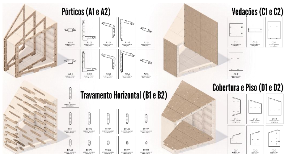
Figura 5. Demonstração das peças existentes nos módulos com suas respectivas planificações.
