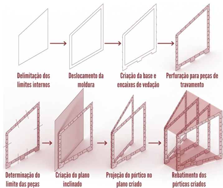
Figura 2. Diagrama apresentando processo de geração da forma.
