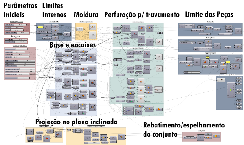
Figura 3. Definição desenvolvida no grasshopper para geração dos pórticos.
