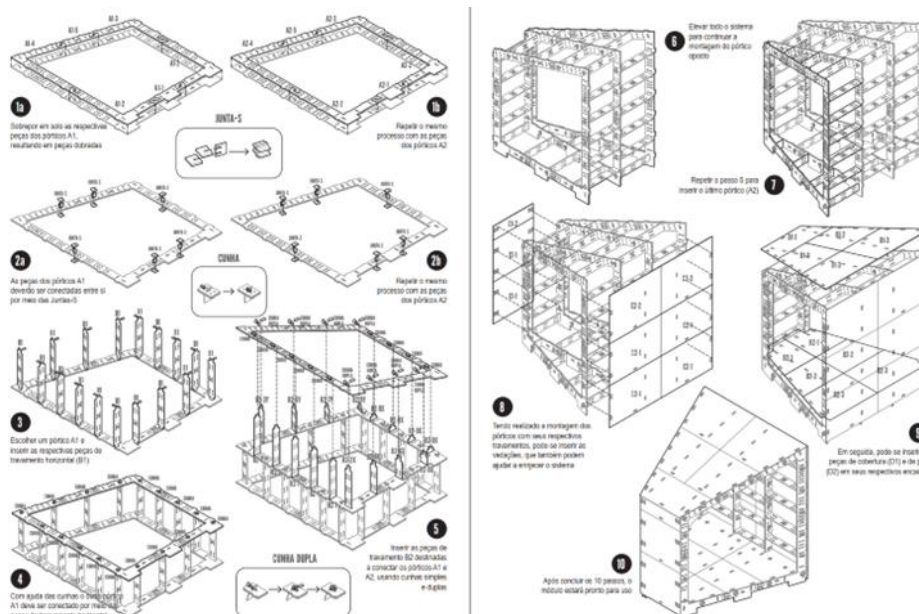
Figura 10. Manual de montagem desenvolvido para o sistema.
