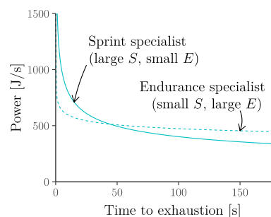
Fig. 3 Role of the speed parameter S and the endurance parameter E
